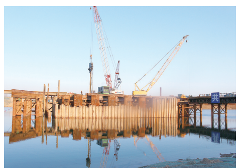
牡丹江路沙河大桥桩基施工现场
